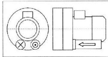
图. 2: 2HB740-HH57(双叶轮规格)
