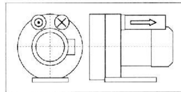
图. 3: 2HB840(双叶轮大流量规格)
