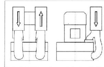
图. 6: 2HB940-BH47(双叶轮大流量规格)
